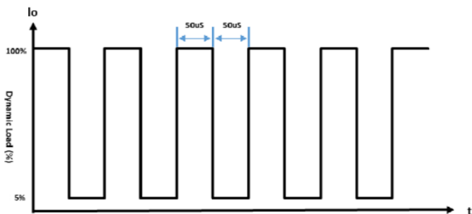
图 5-2. 动态负载
