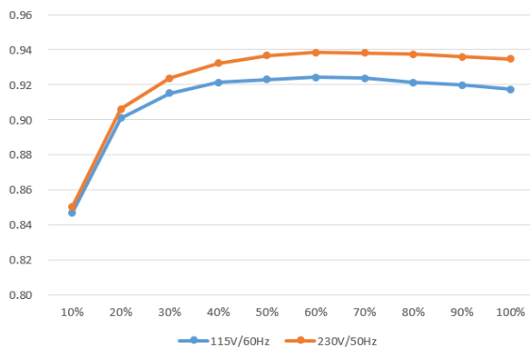
图 1. 12 V (max. 200 W) 机种典型效率曲线
